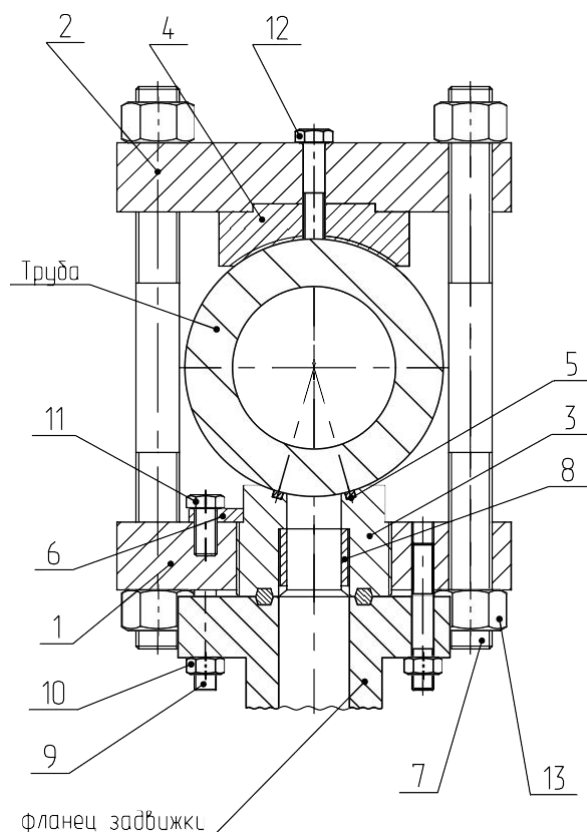
Рисунок 2 – Монтаж приспособления на трубе при помощи хомута
